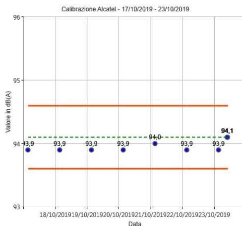
Figura 31 Calibrazioni check postazione Alcatel
