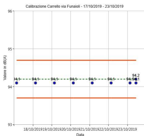
Figura 26: Calibrazioni check postazione Carrello Via Funaioli
