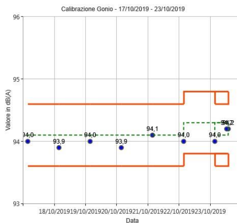
Figura 30: Calibrazioni check postazione Gonio
