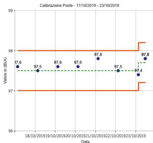
Figura 29: Calibrazioni check postazione Poste
