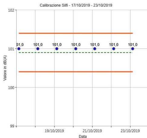
Figura 28: Calibrazioni check postazione Silfi
