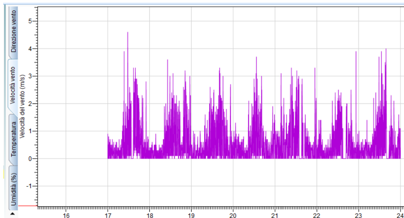
Figura 23: Grafico della velocità del vento acquisita dalla centralina Silfi
