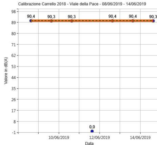
Figura 27: Calibrazioni check postazione Carrello Via della Pace
