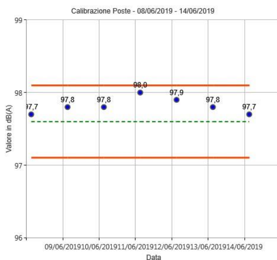
Figura 29: Calibrazioni check postazione Poste
