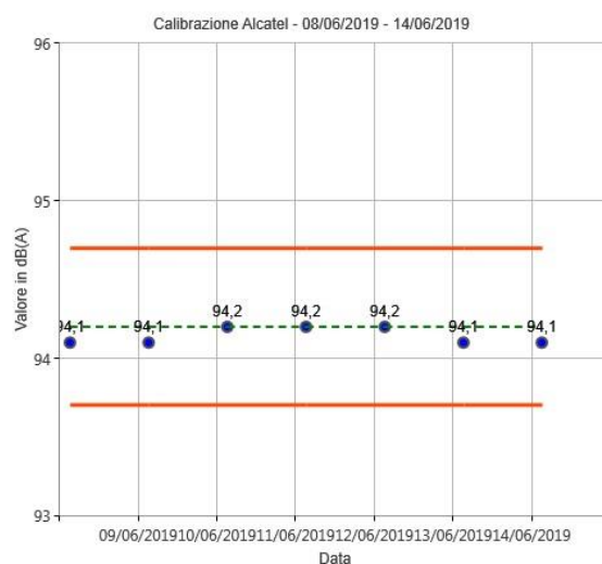
Figura 31 Calibrazioni check postazione Alcatel
