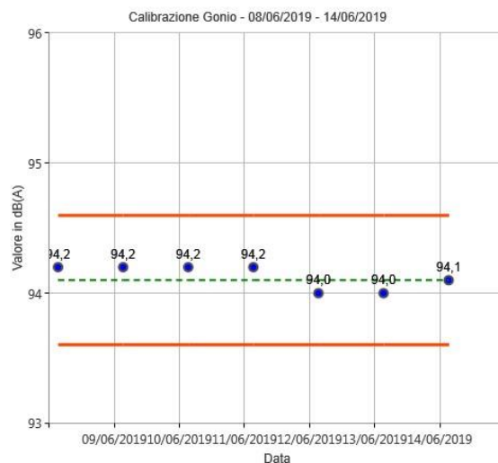
Figura 30: Calibrazioni check postazione Gonio
