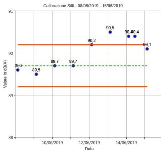
Figura 28: Calibrazioni check postazione Silfi
