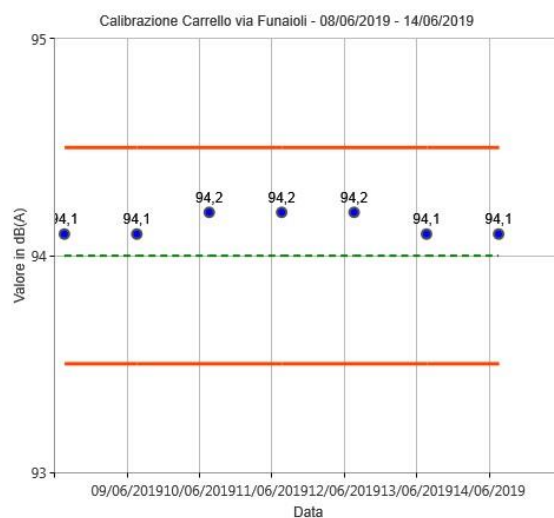
Figura 26: Calibrazioni check postazione Carrello Via Funaioli
