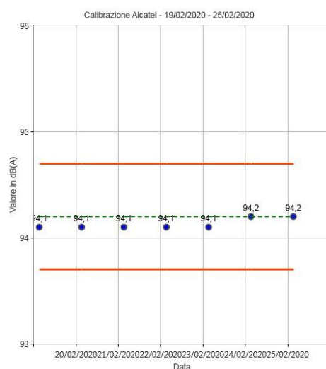
Figura 31 Calibrazioni check postazione Alcatel
