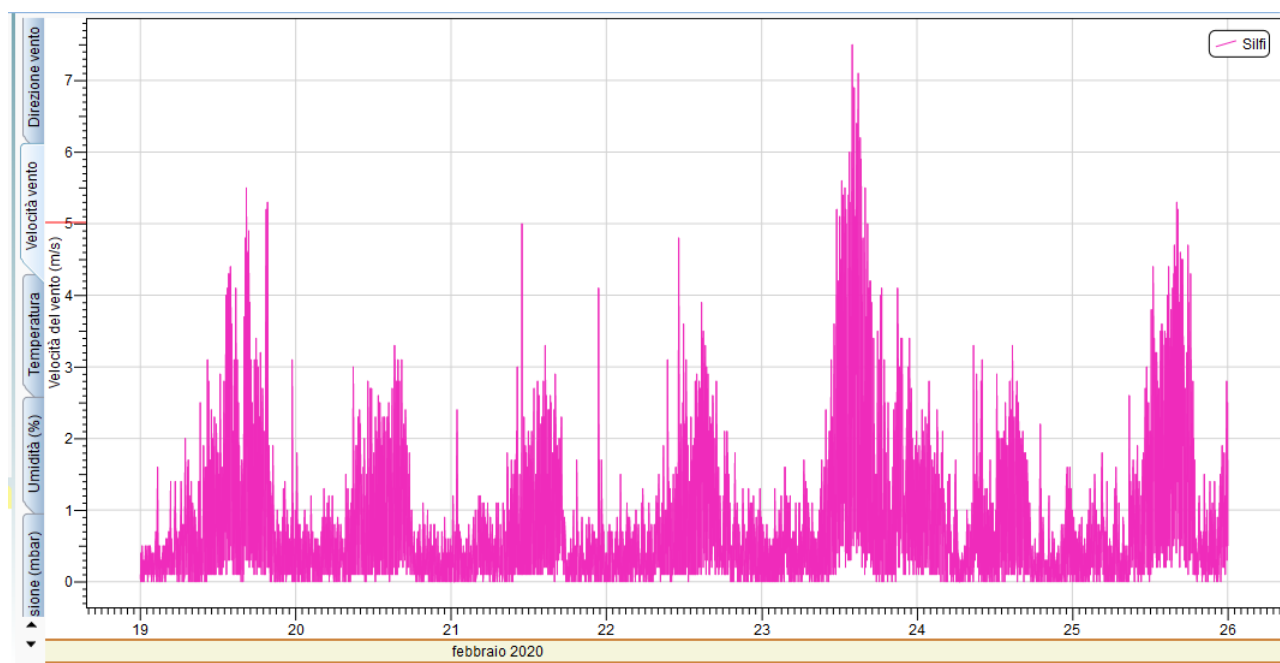
Figura 25: Grafico della velocità del vento acquisita dalla centralina Silfi
