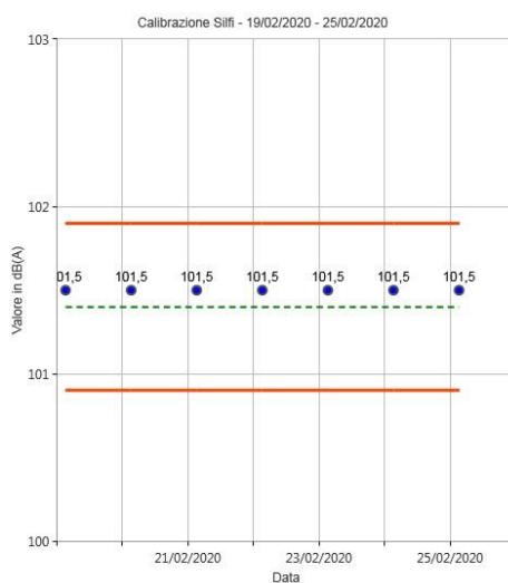
Figura 28: Calibrazioni check postazione Silfi
