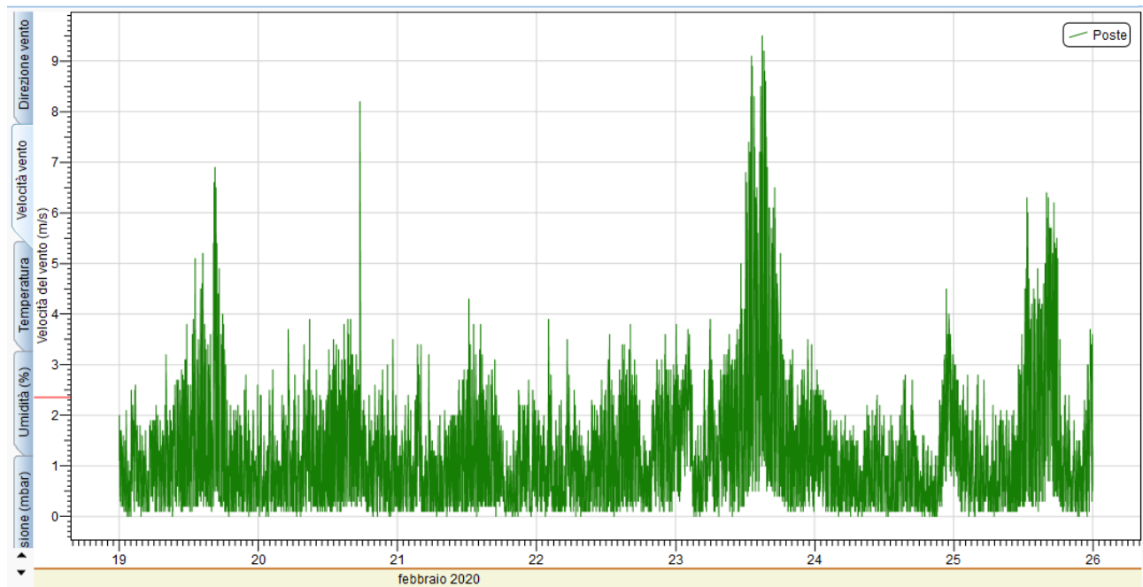
Figura 23: Grafico della velocità del vento acquisita dalla centralina POSTE
