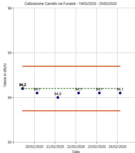
Figura 28: Calibrazioni check postazione Carrello Via Funaioli
