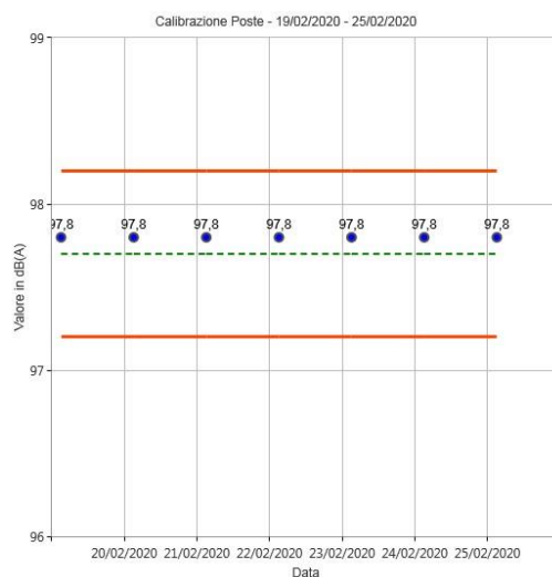
Figura 29: Calibrazioni check postazione Poste
