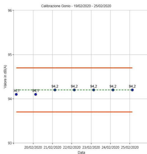
Figura 30: Calibrazioni check postazione Gonio
