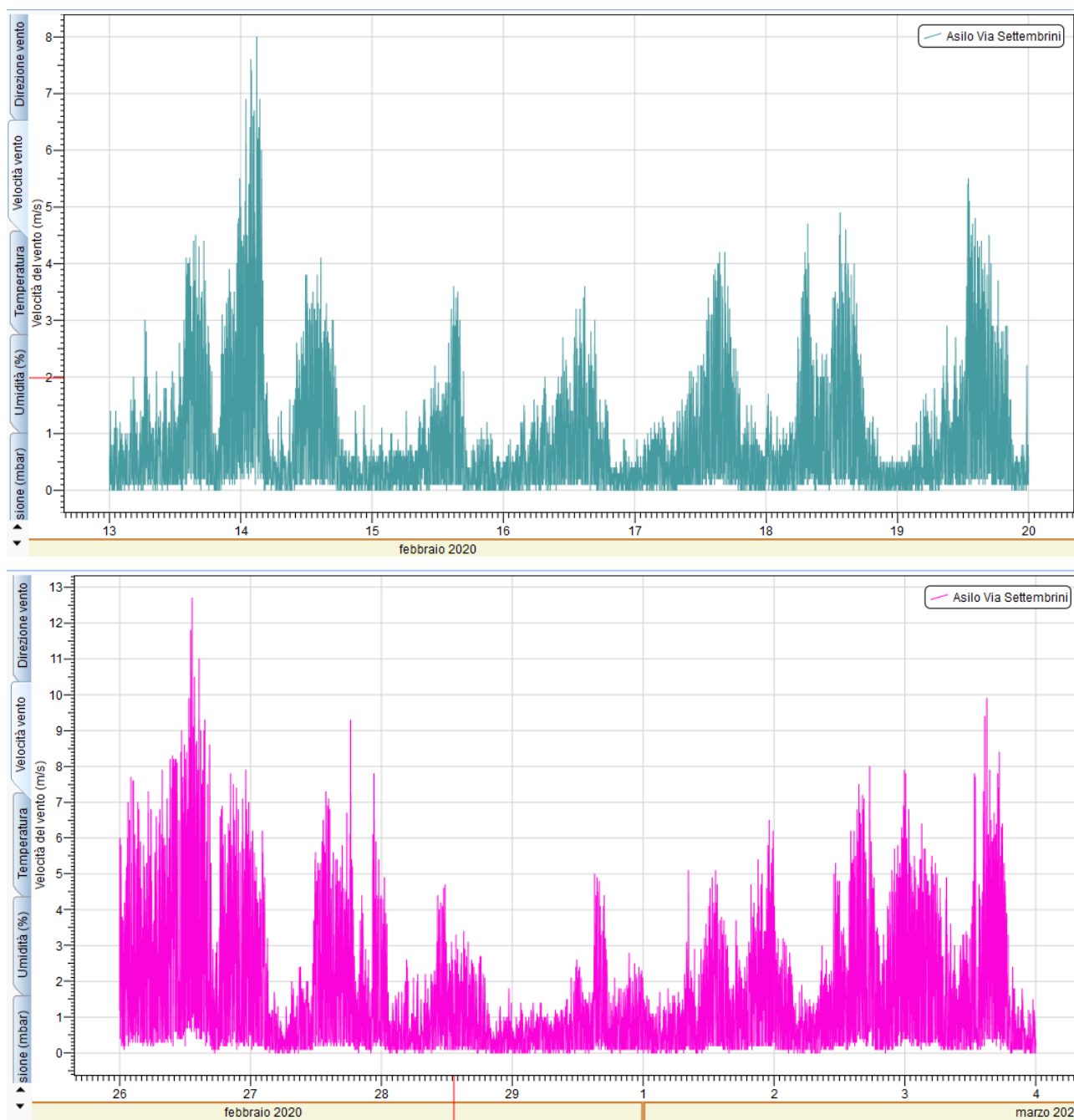
Figura 22: Grafico della velocità del vento acquisita dalla centralina Asilo Via Settembrini per entrambe le settimane prese in esame
