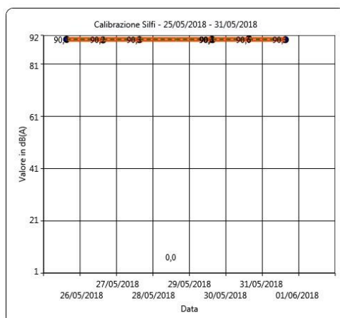
Figura 33: Calibrazioni check postazione Silfi
