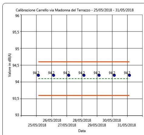
Figura 37: Calibrazioni check postazione Carrello Via Madonna del Terrazzo
