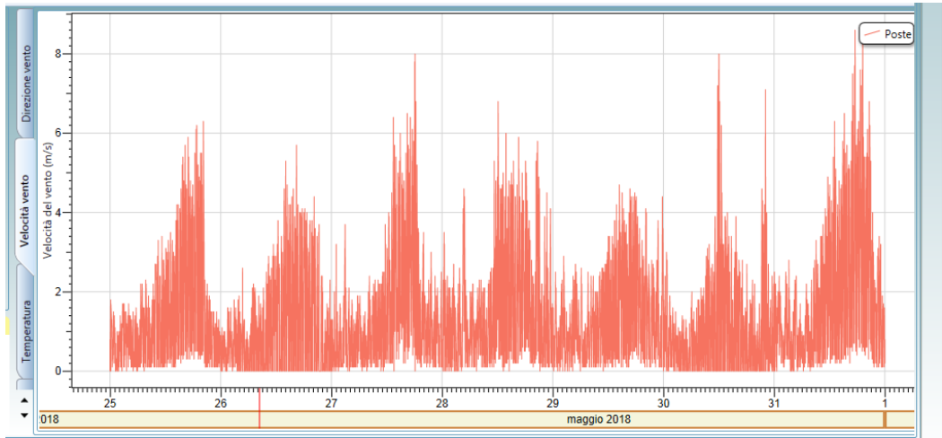
Figura 23: Grafico della velocità del vento acquisita dalla centralina POSTE
