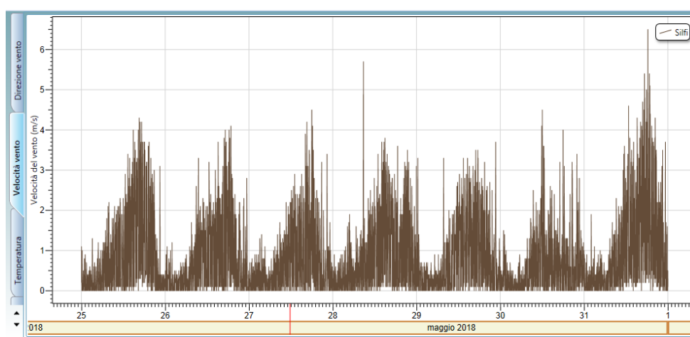
Figura 25: Grafico della velocità del vento acquisita dalla centralina Silfi
