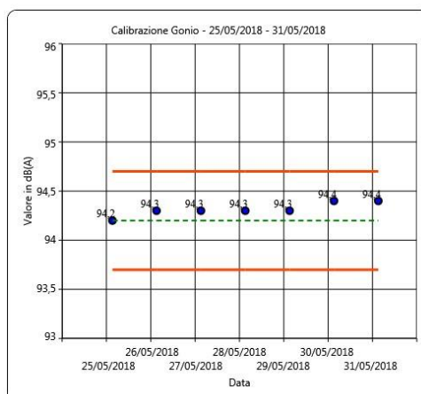
Figura 35: Calibrazioni check postazione Gonio
