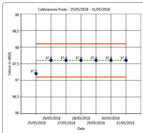
Figura 34: Calibrazioni check postazione Poste
