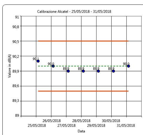
Figura 36: Calibrazioni check postazione Alcatel
