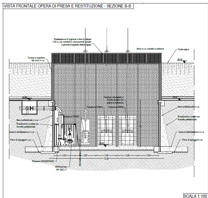
Figura 8-5: Opera di restituzione
