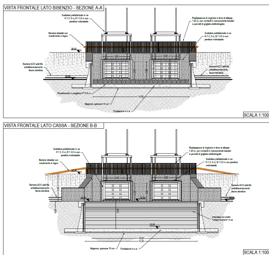
Figura 8-4: Opera di presa tipo
