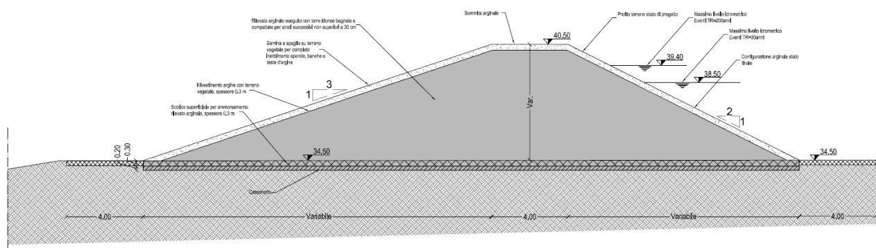
Figura 8-3: Sezione tipologica arginature tratto B.
