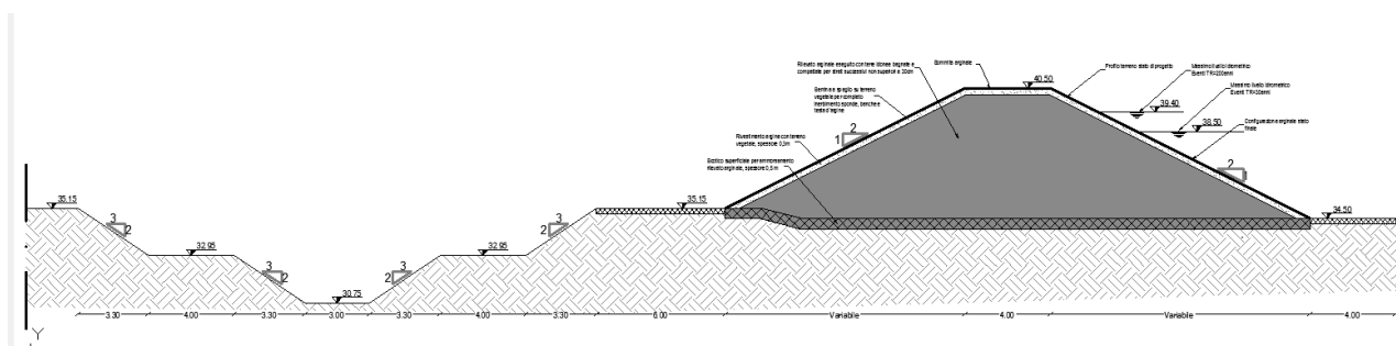
Figura 8-2: Sezione tipologica arginature tratto A.
