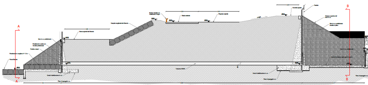
Figura 8-6: Opera di derivazione dal F. Bisenzio
