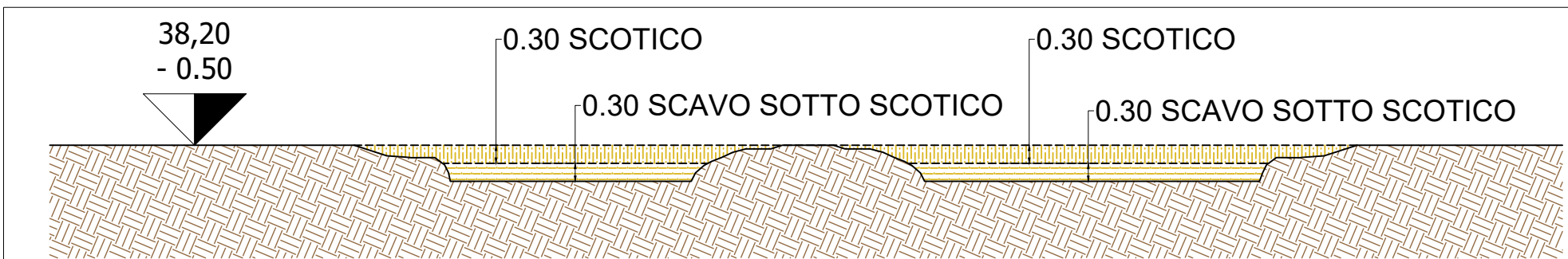
SEZIONE A-A' PROFILO DI SCAVO - scala lunghezze 1:200 - scala altezze 1:100
