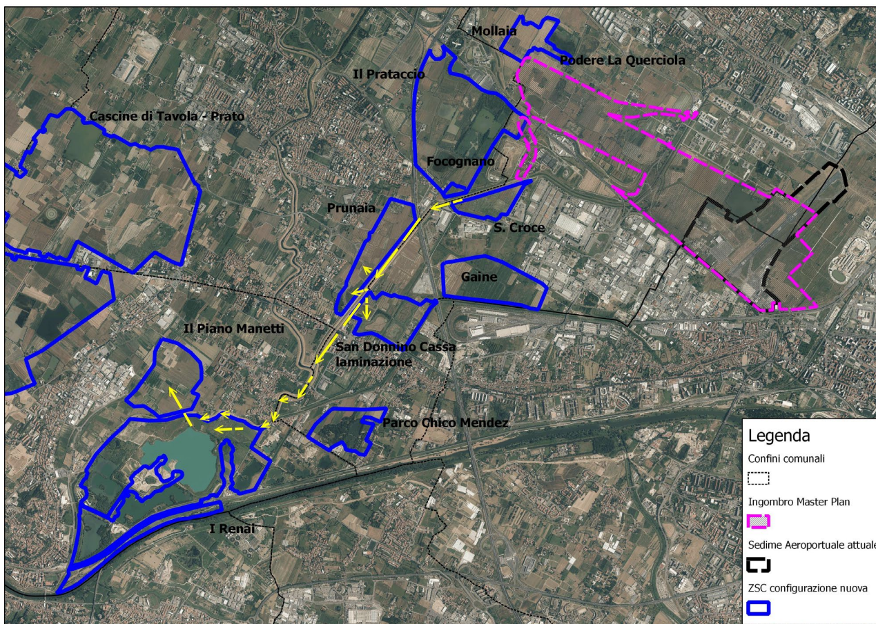
Figura 7 - Santa Croce: connettività ecologica a scala di paesaggio.
