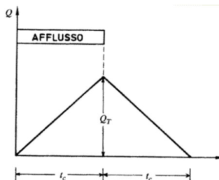
Figure 3 Idrogramma Metodo Razionale
