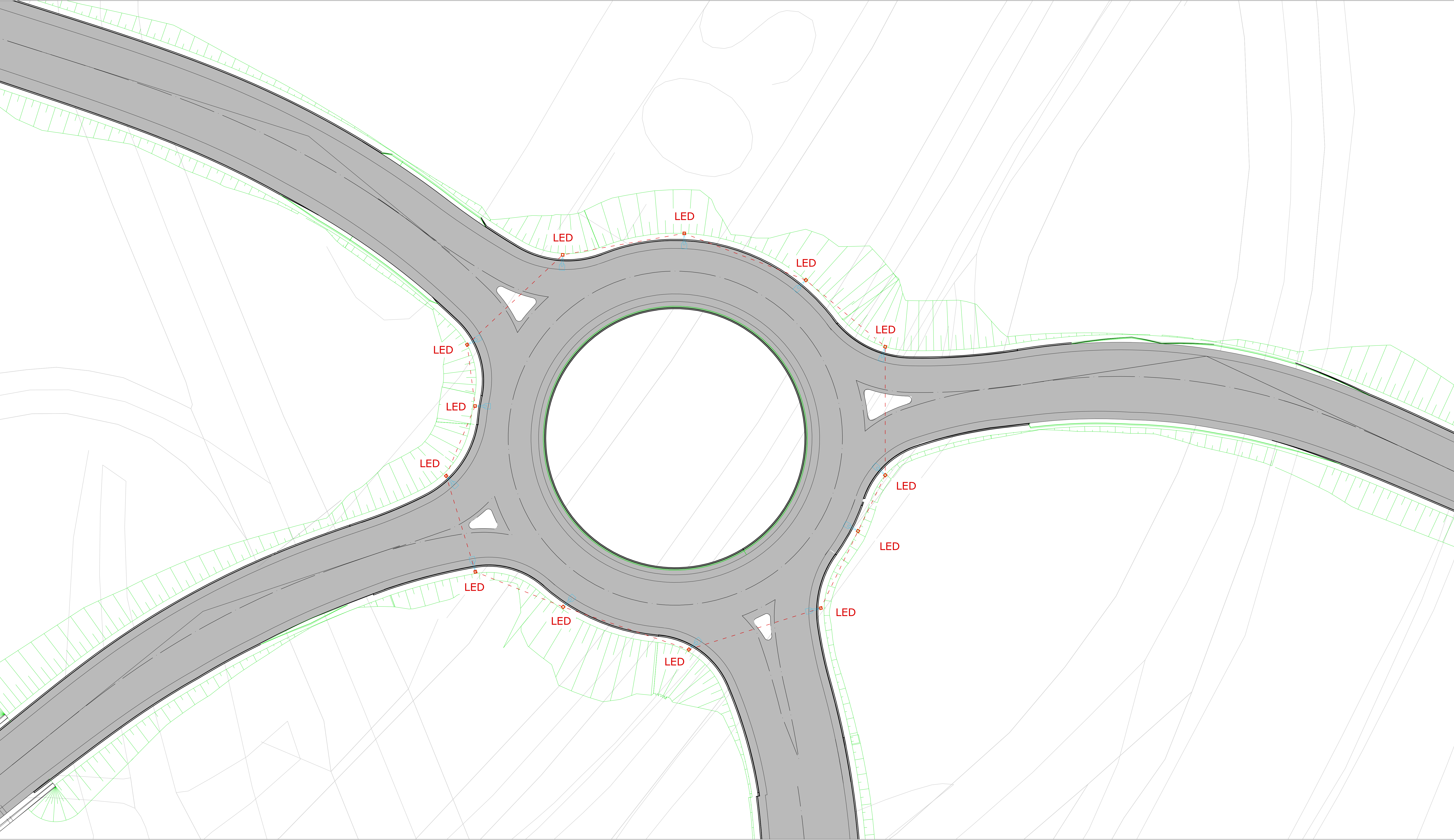
Planimetria Posizionamento Apparecchiature e Impianti Elettrici Rotatoria B Scala 1:200
